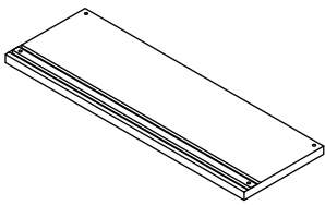
② 地板 ×1
